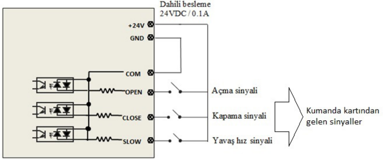
Şekil 2 Dâhili 24V DC Besleme İle Bağlantı
