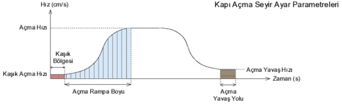
Şekil 9 Kapı Açma Grafiği
